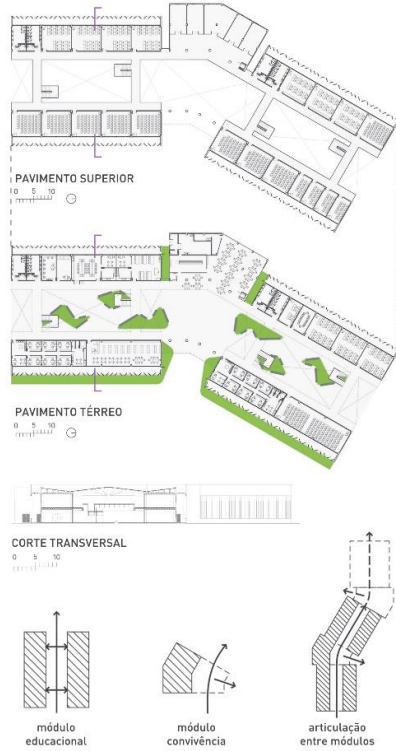
Figure 2. Desenhos técnicos, diagramas, fachadas e área de convivência. Rede Arquitetos e Croquis Projetos.
