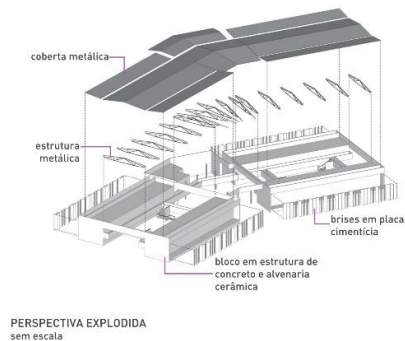
Figure 3. Diagrama de estruturas, fachadas e área de estar e circulação. Rede Arquitetos e Croquis Projetos.
